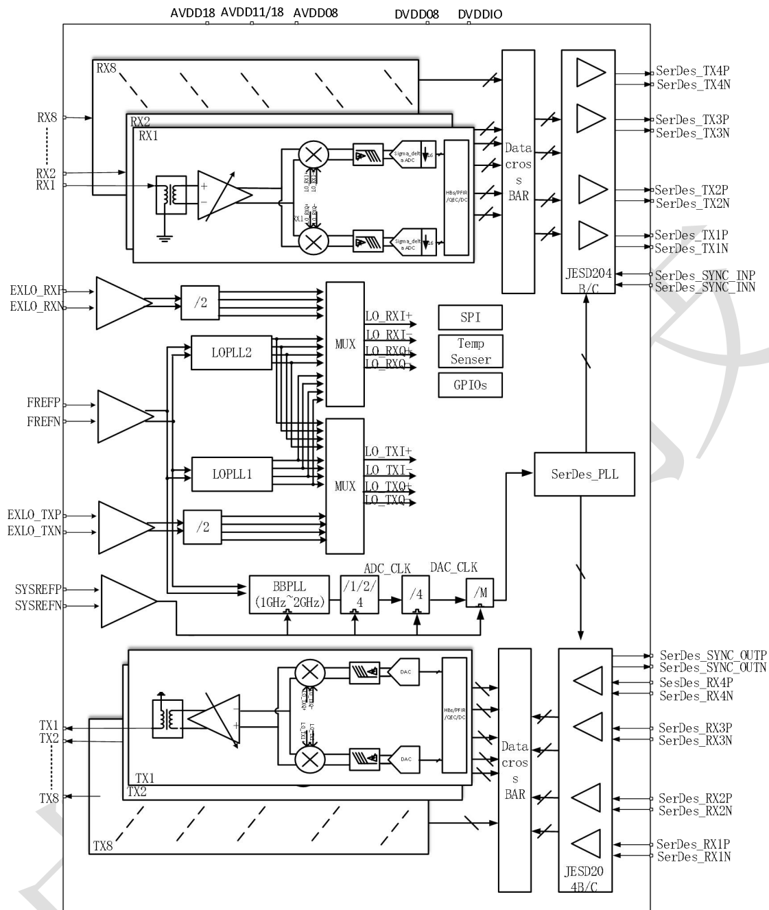
图 1 CX9840A/CX9840AN 功能框图
