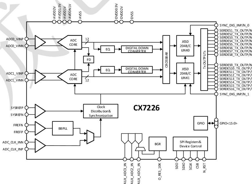
图 1 CX7226/CX7226N 功能框图
