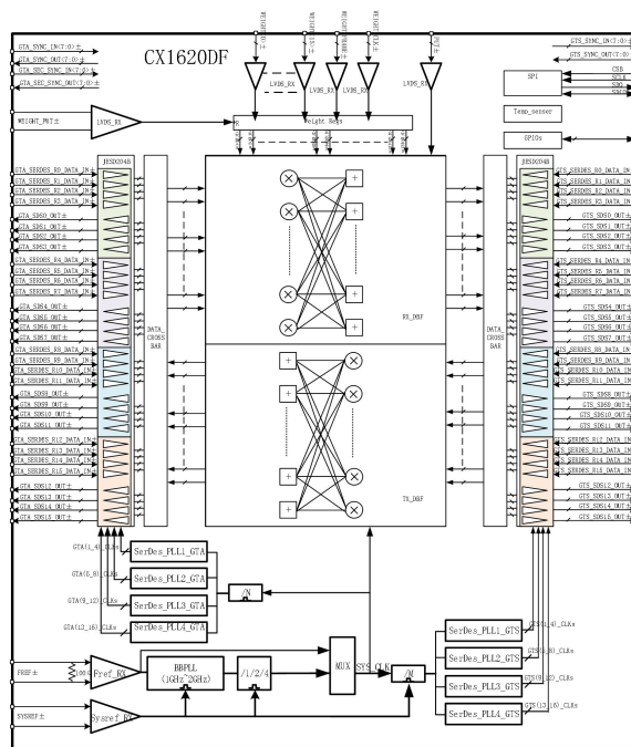
图 1 CX1620DF/CX1620DFN 功能框图
