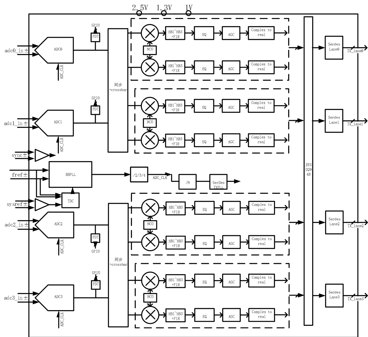
CX7442A/CX7442AN 功能框图
