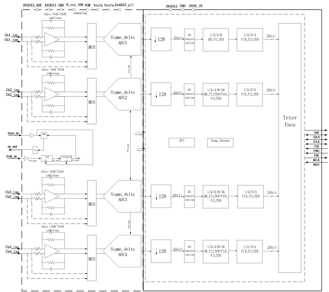
CX74E1/ CX74E1N 器件功能框图：
