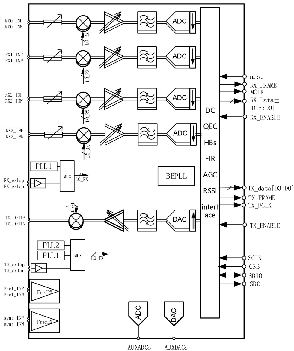
CX9450/CX9450N 功能框图
