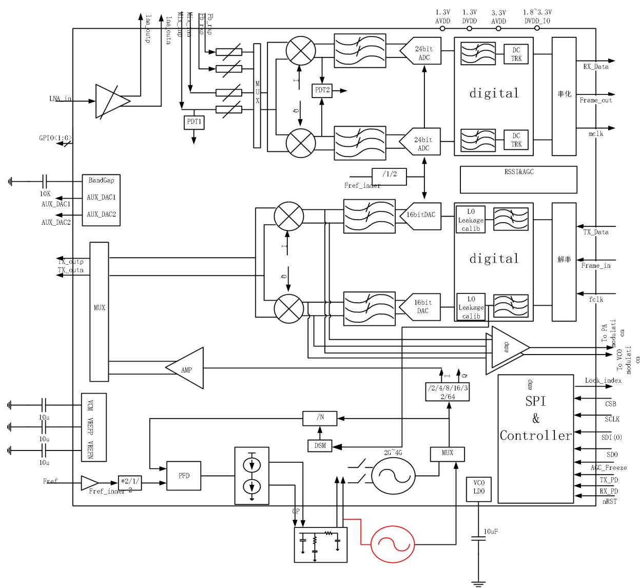
CX91E1 功能框图
