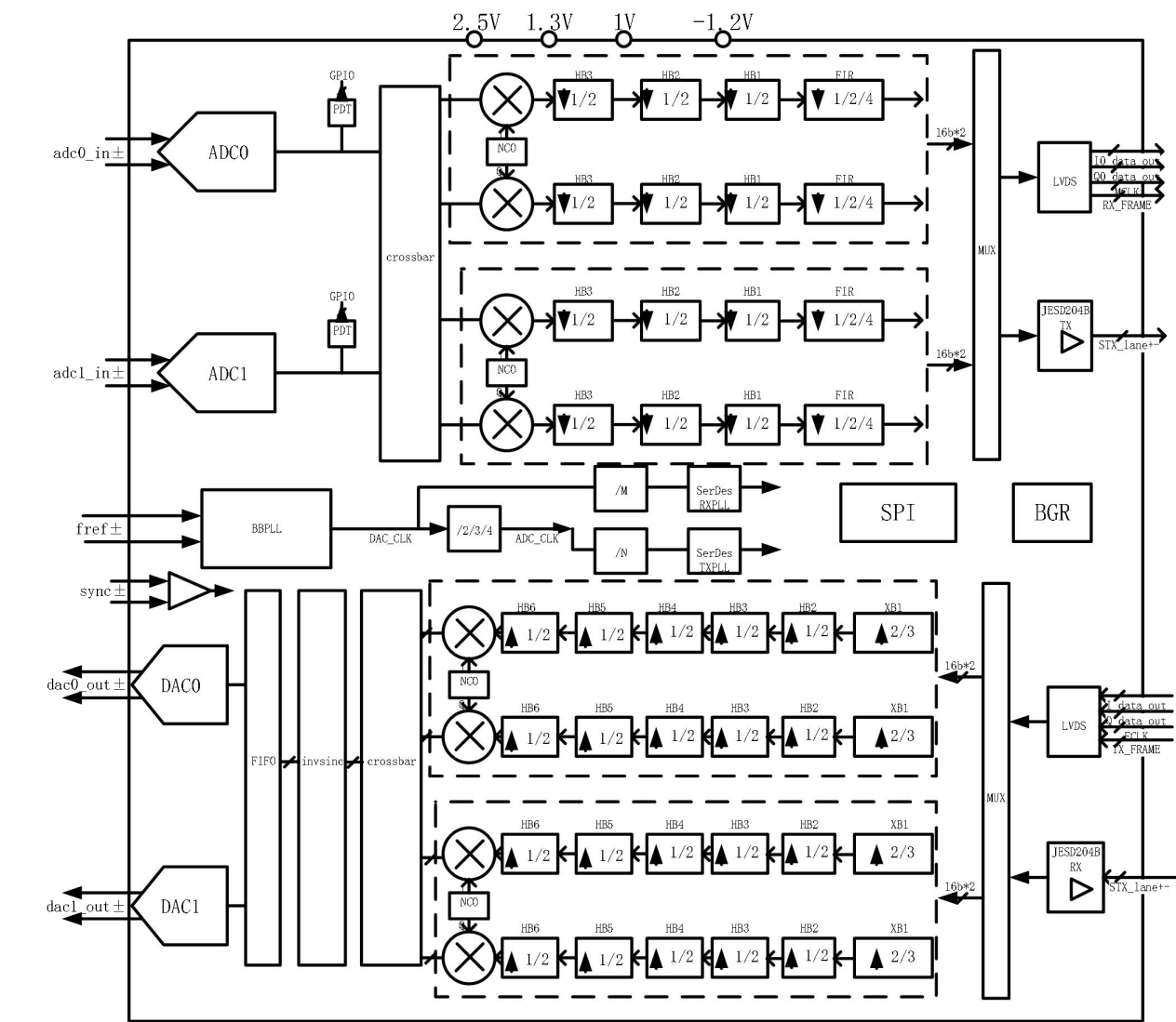
CX8142/CX8142N 功能框图
