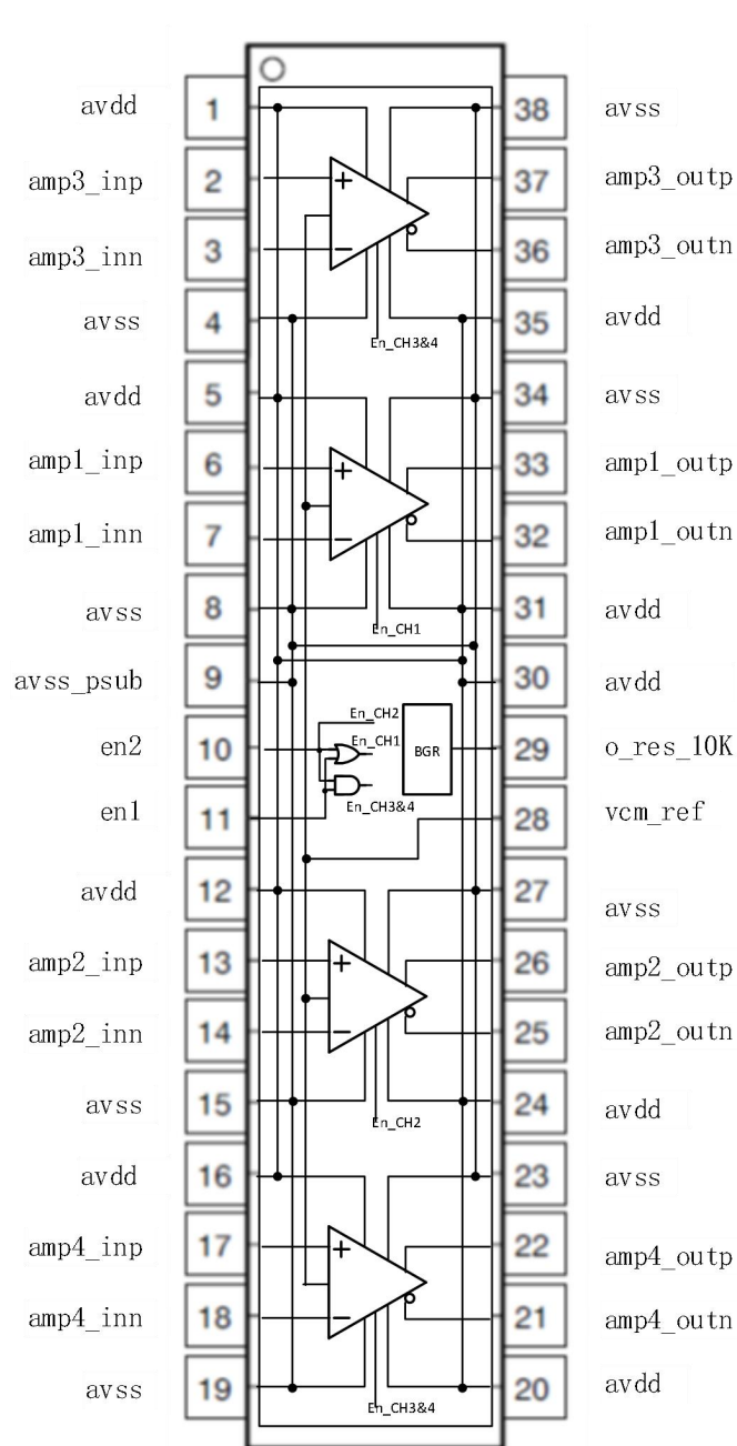
CX2402/CX2402N 封装示意图
