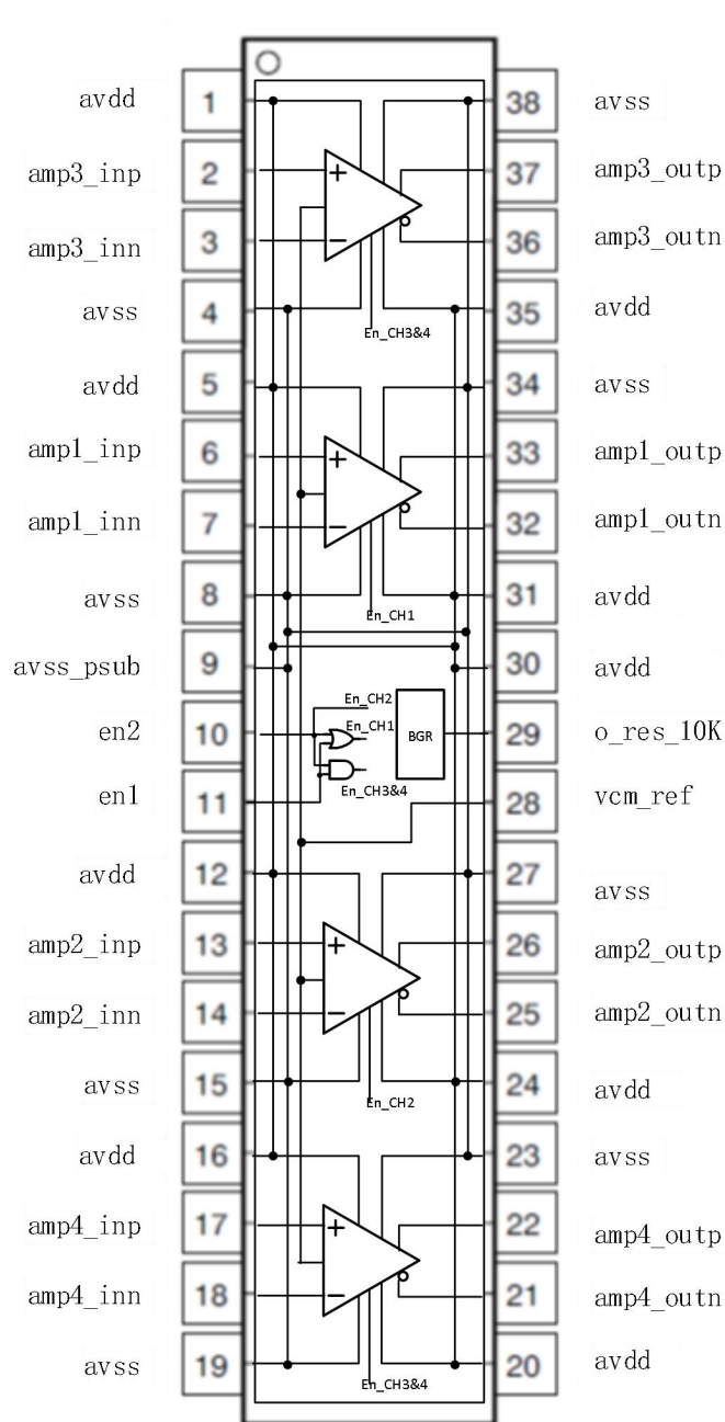
CX2401/CX2401N 封装示意图
