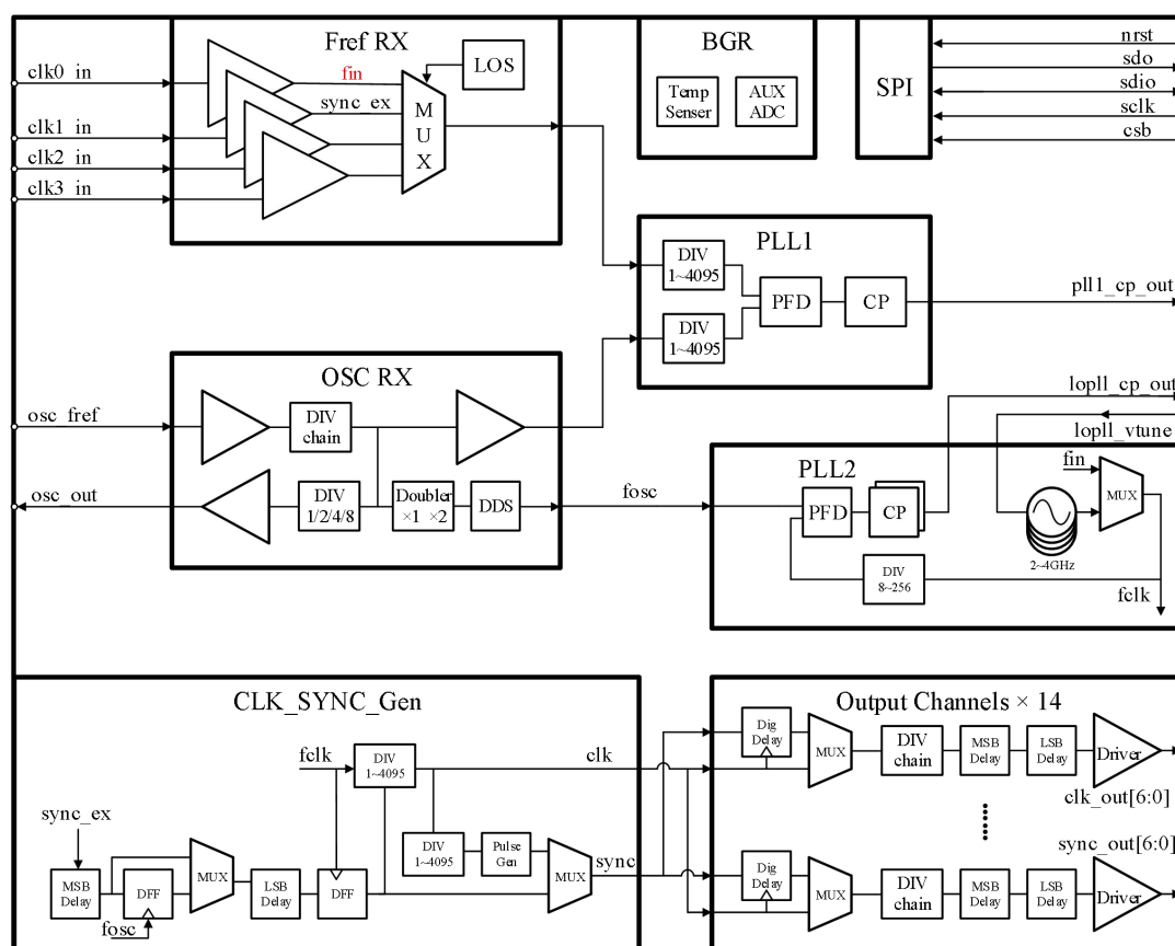
CX4E04A/CX4E04AN 功能框图
