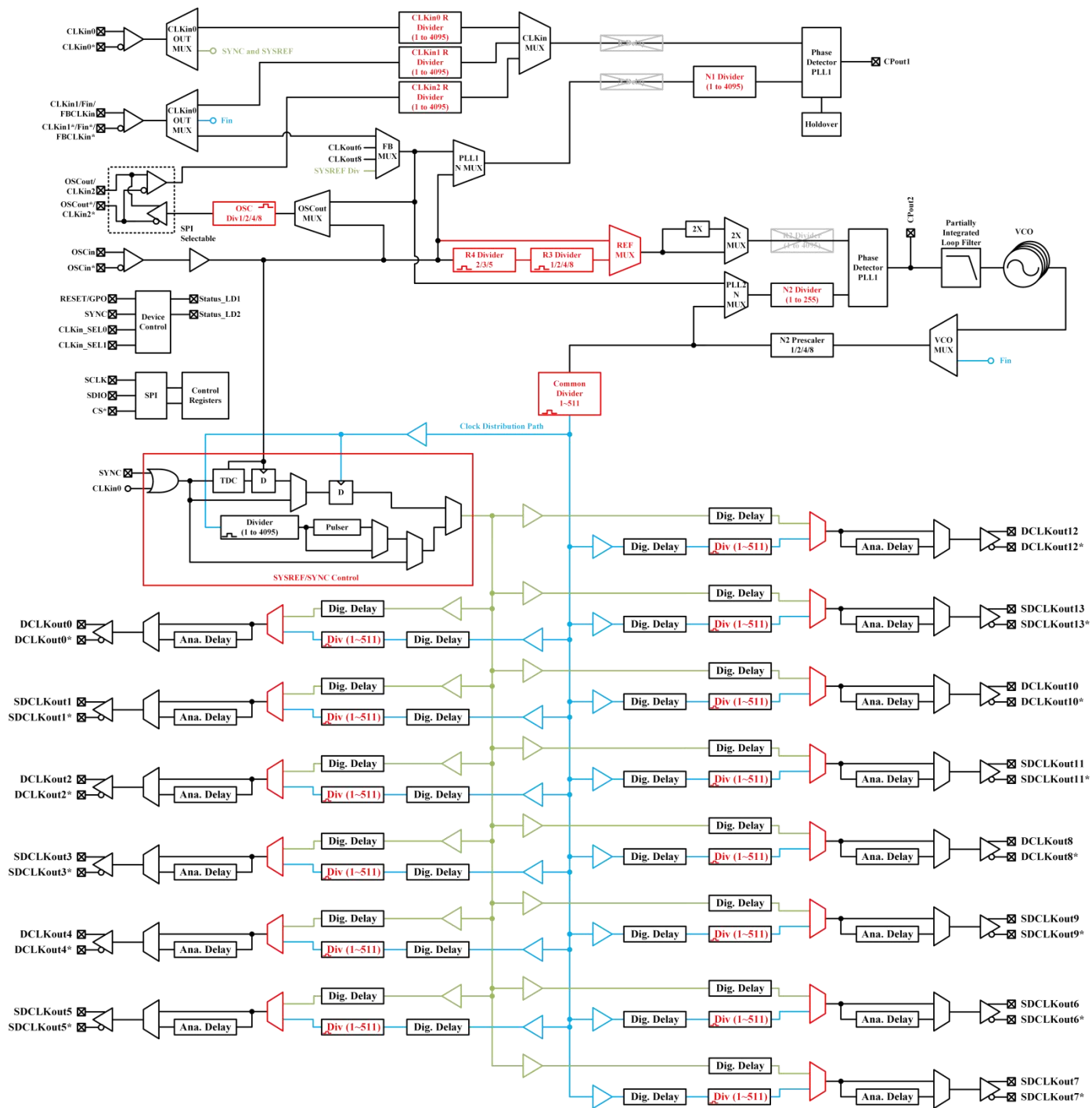
CX4E06A/ CX4E06AN 器件功能框图:
